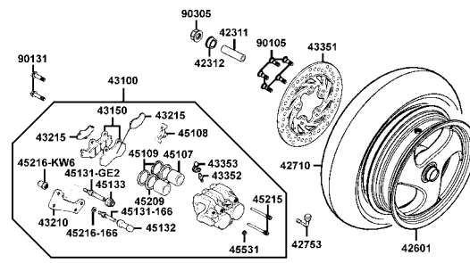
F8 後輪 -77- Rear Wheel
